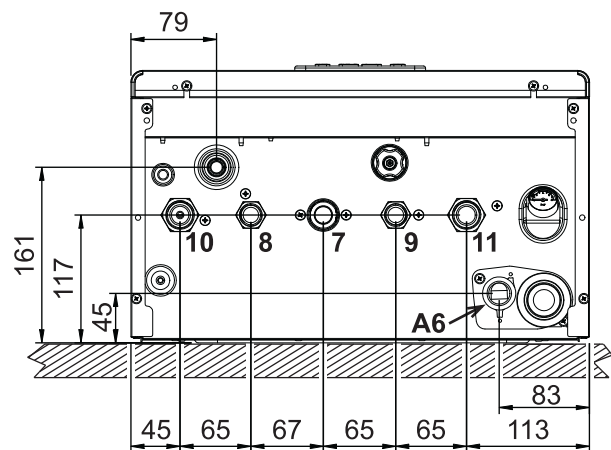
fig. 35- Vista inferior
