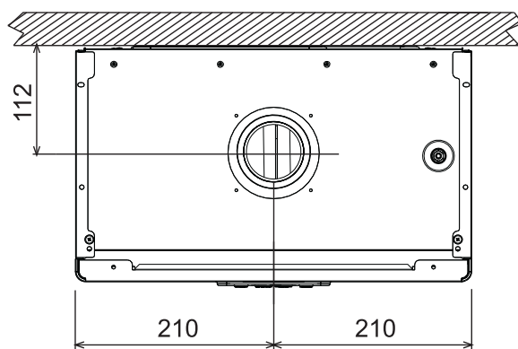
fig. 34- Vista superior
