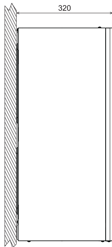
fig. 37- Vista lateral
