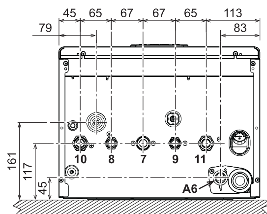
fig. 39- Vista inferior
