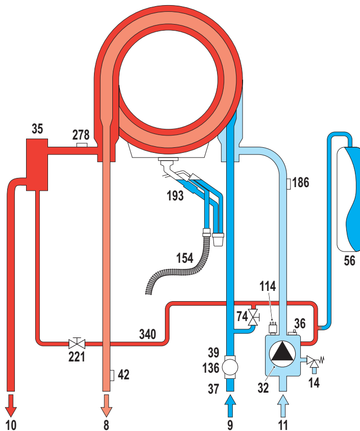
fig. 27 - Circuito hidráulico
