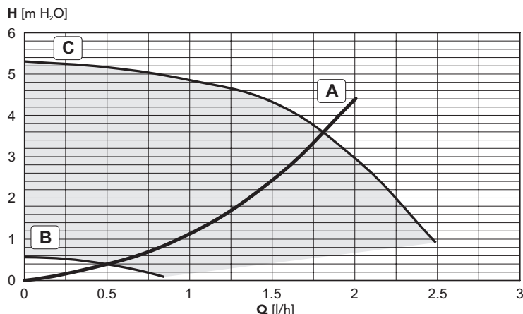
fig. 28 - Pérdida de carga/altura manométrica bomba
