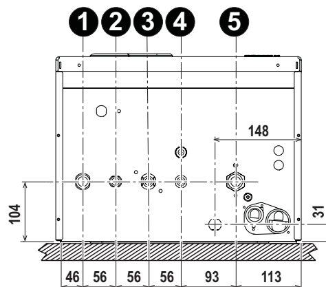
fig. 13 - Conexiones hidráulicas
