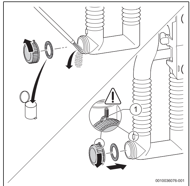
Fig. 47 Limpiar el sifón de condensados
