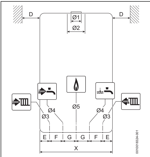
Fig. 3 Vista frontal
