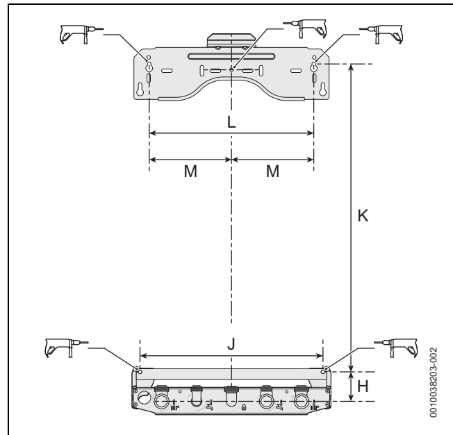
Fig. 4 Clip de fijación suspendido y puntos de sujeción
