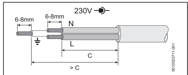
Fig. 27 Suministro de corriente (cables de corriente), preparación
