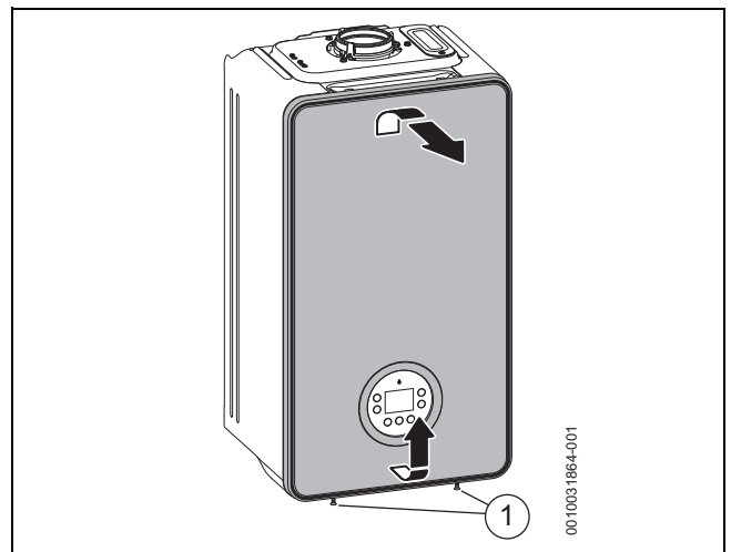
Fig. 32 Retirar la carcasa frontal
