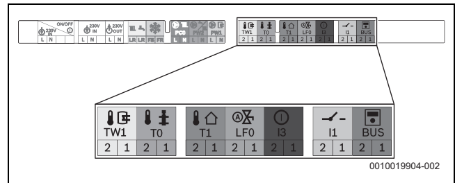
Fig. 30 Bornera de baja tensión (cables de señales)
