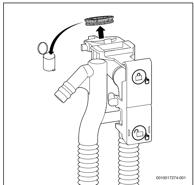
Fig. 48 Retirar la junta en la parte superior del sifón de condensados
