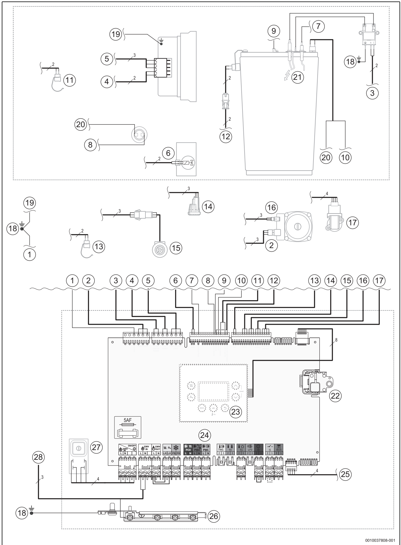
Fig. 66 Cableado eléctrico
