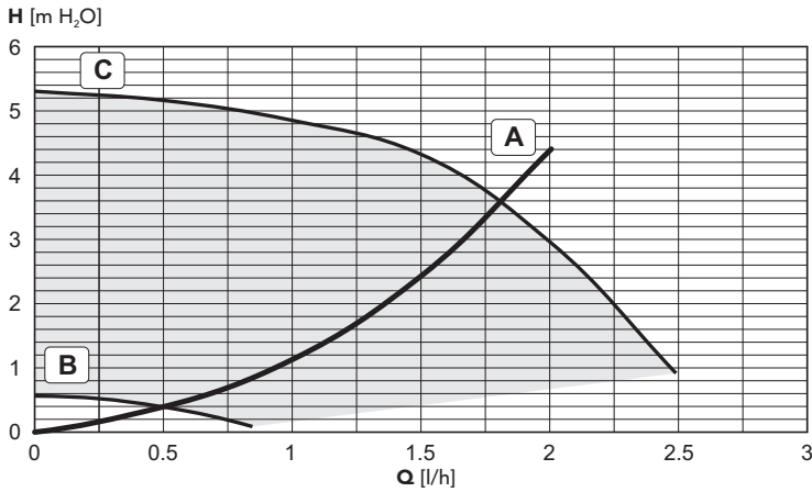
fig. 28 - Pérdida de carga/altura manométrica bomba SUPERLATIVE CONDENS 25C
