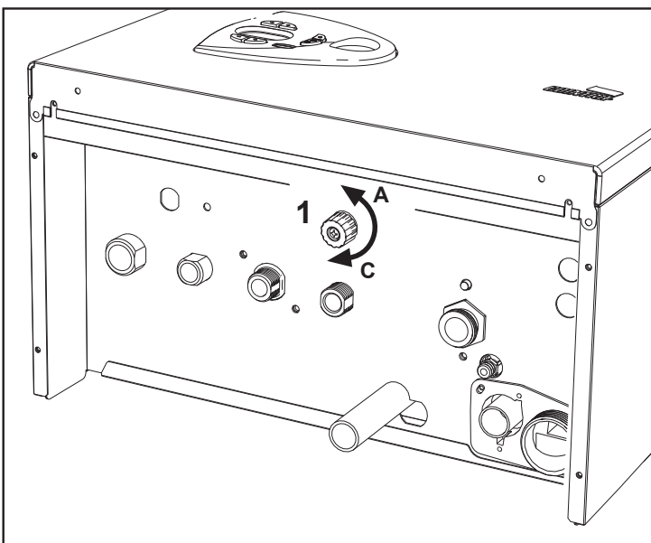
fig. 12 - Llave de llenado
