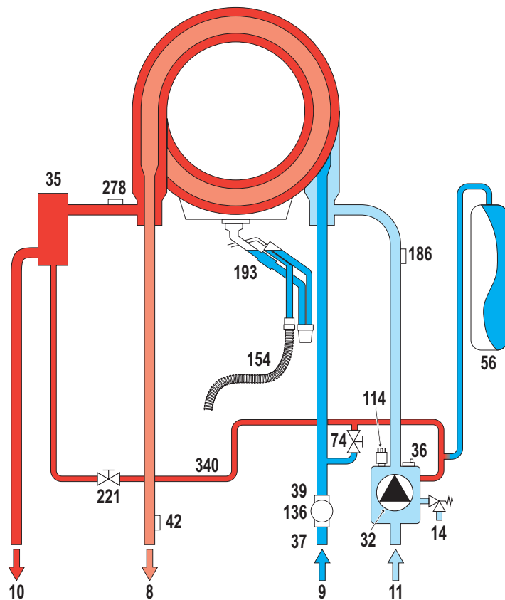
fig. 27 - Circuito hidráulico
