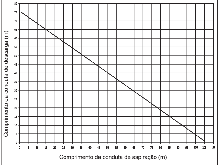
COMPRIMENTO RECTILÍNEO Ø 80
