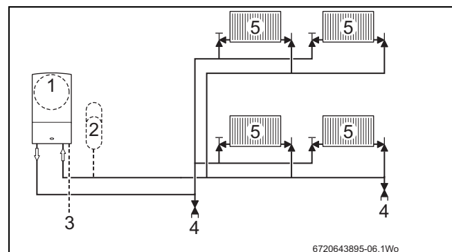
Fig. 6 Sistema cerrado
