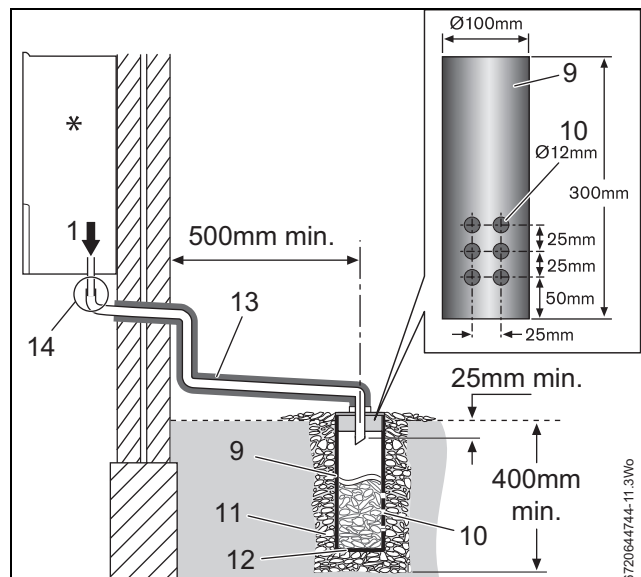
Fig. 14 Pozo absorbente
