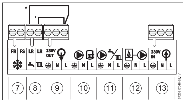
Fig. 53 Conectores de tensión de red
