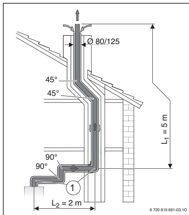
Fig. 29 Situación de montaje de una evacuación de gases según C 33
