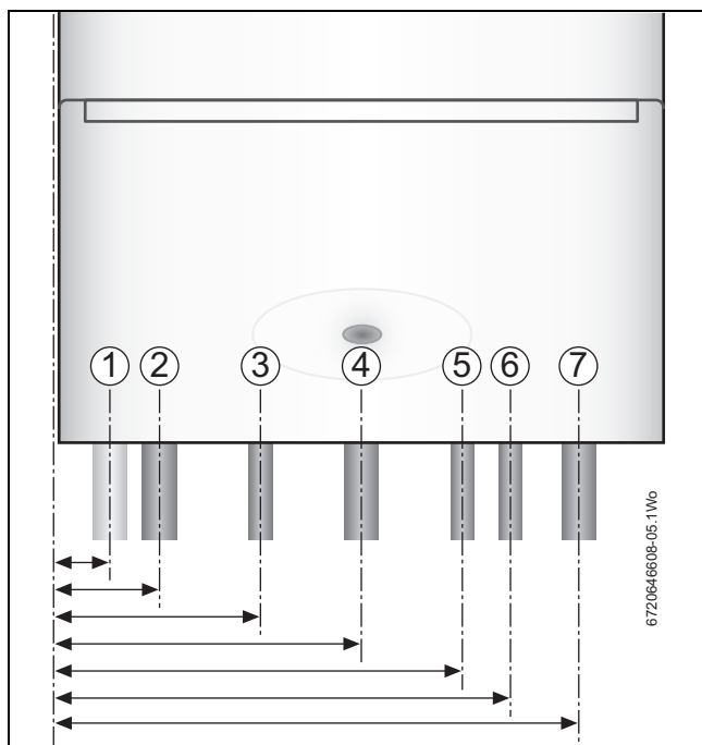
Fig. 18 Distancias y diámetros de los tubos
