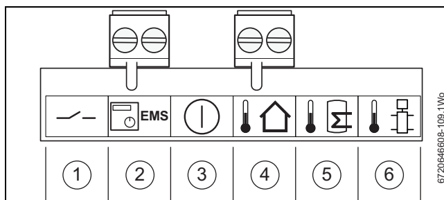
Fig. 52 Conectores de baja tensión
