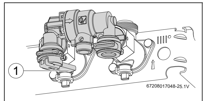
Fig. 63 Grupo de llenado
