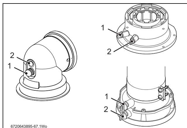
Fig. 74 Puntos de análisis de aire/gases
