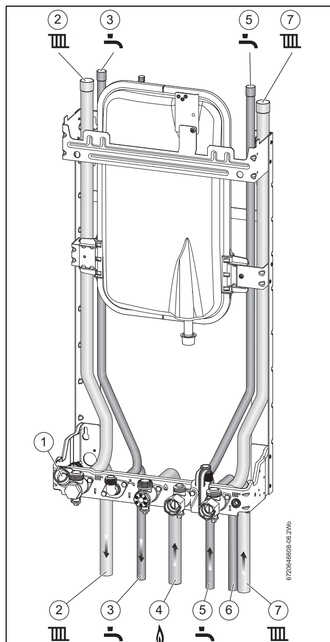
Fig. 19 Tuberías
