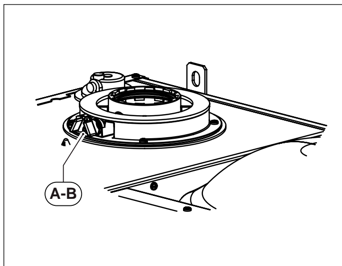
Fig. 19 Posición tapones
