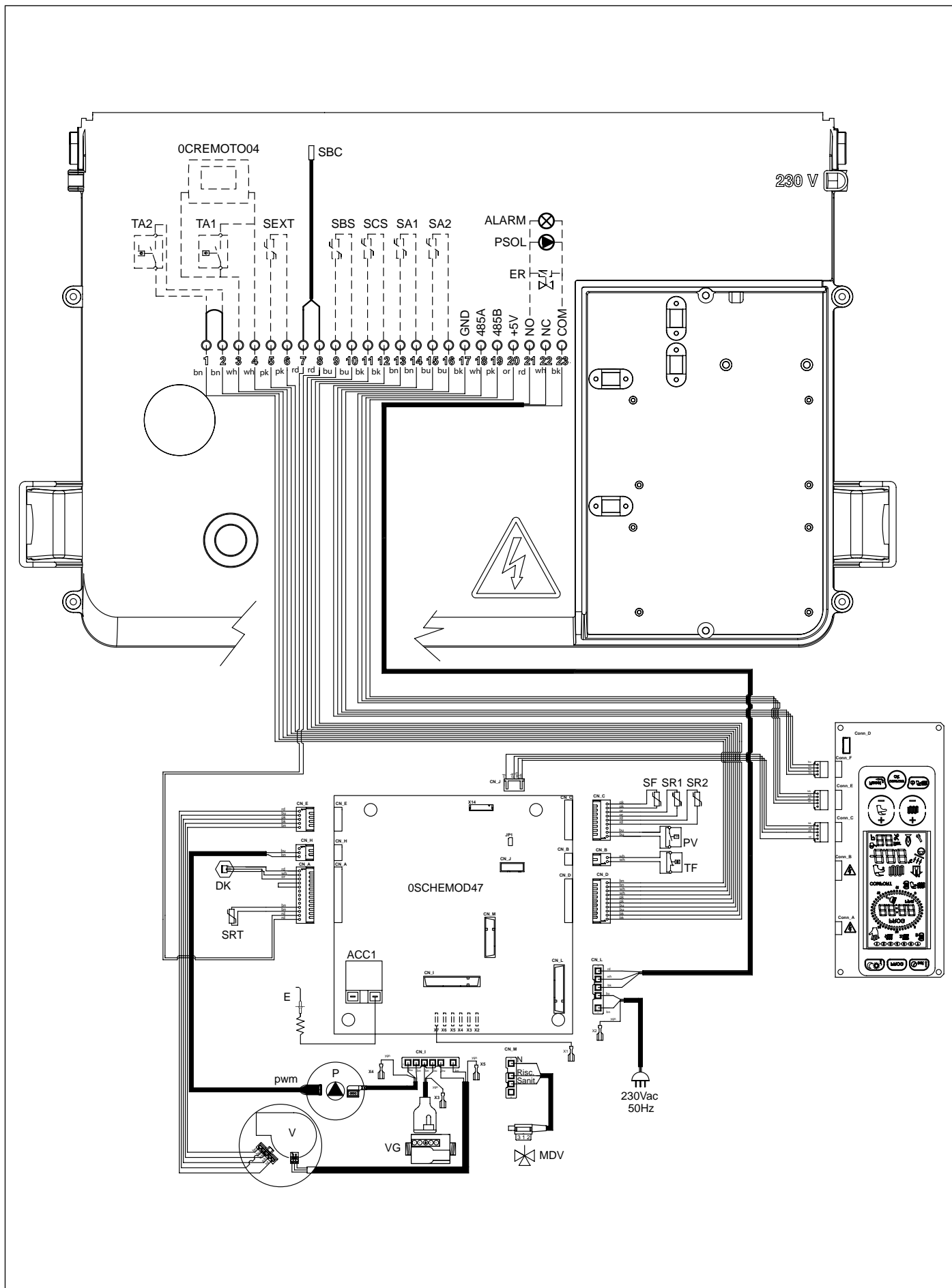
Fig. 25 Esquema eléctrico
