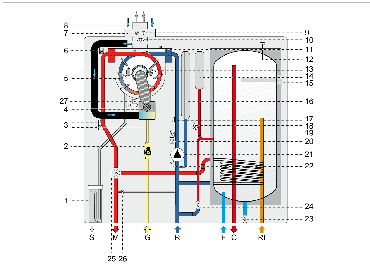
Fig. 5 Esquema hidráulico
