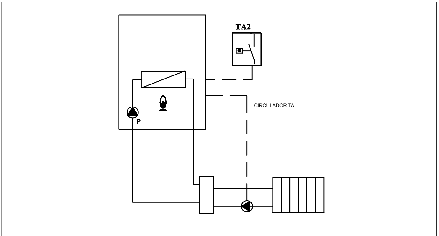
Fig. 30 Relé con pedido (P17=3)
