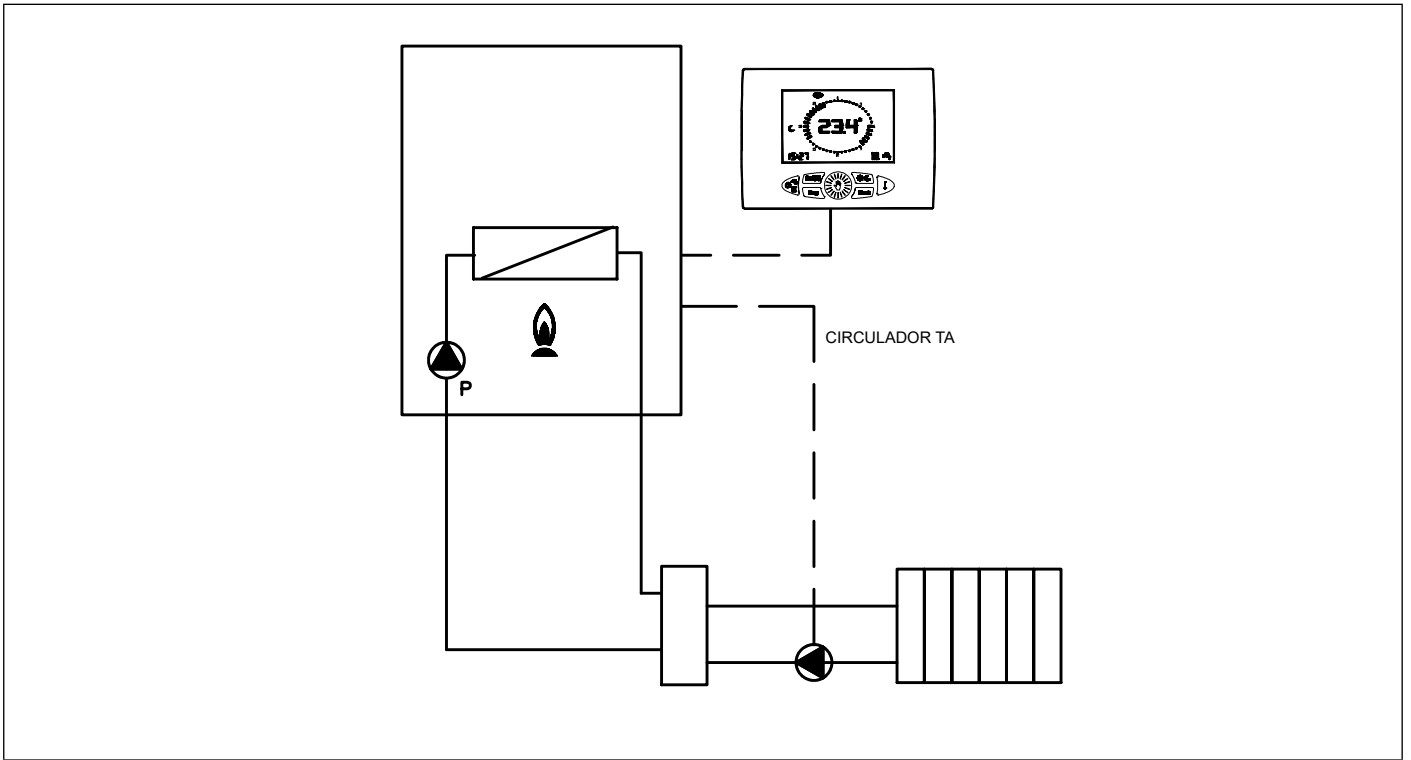
Fig. 29 Relé con pedido a distancia (P17=1)
