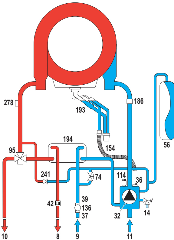
fig. 27 - Circuito hidráulico
