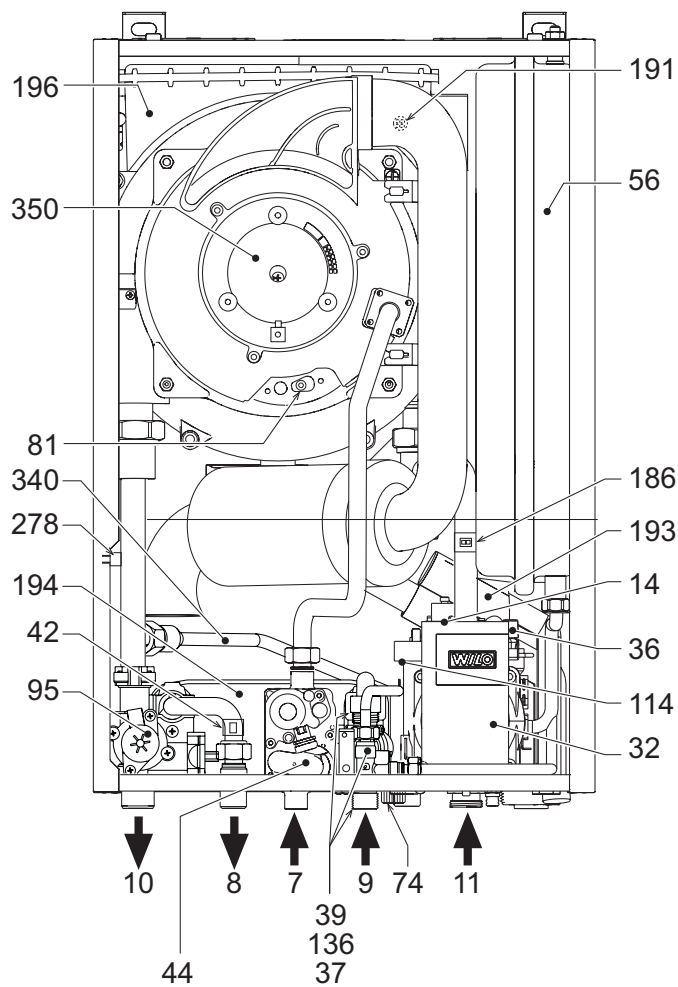
fig. 26 - Vista general
