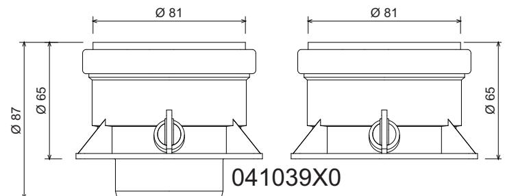
fig. 18 - Accesorio inicial para conductos separados
